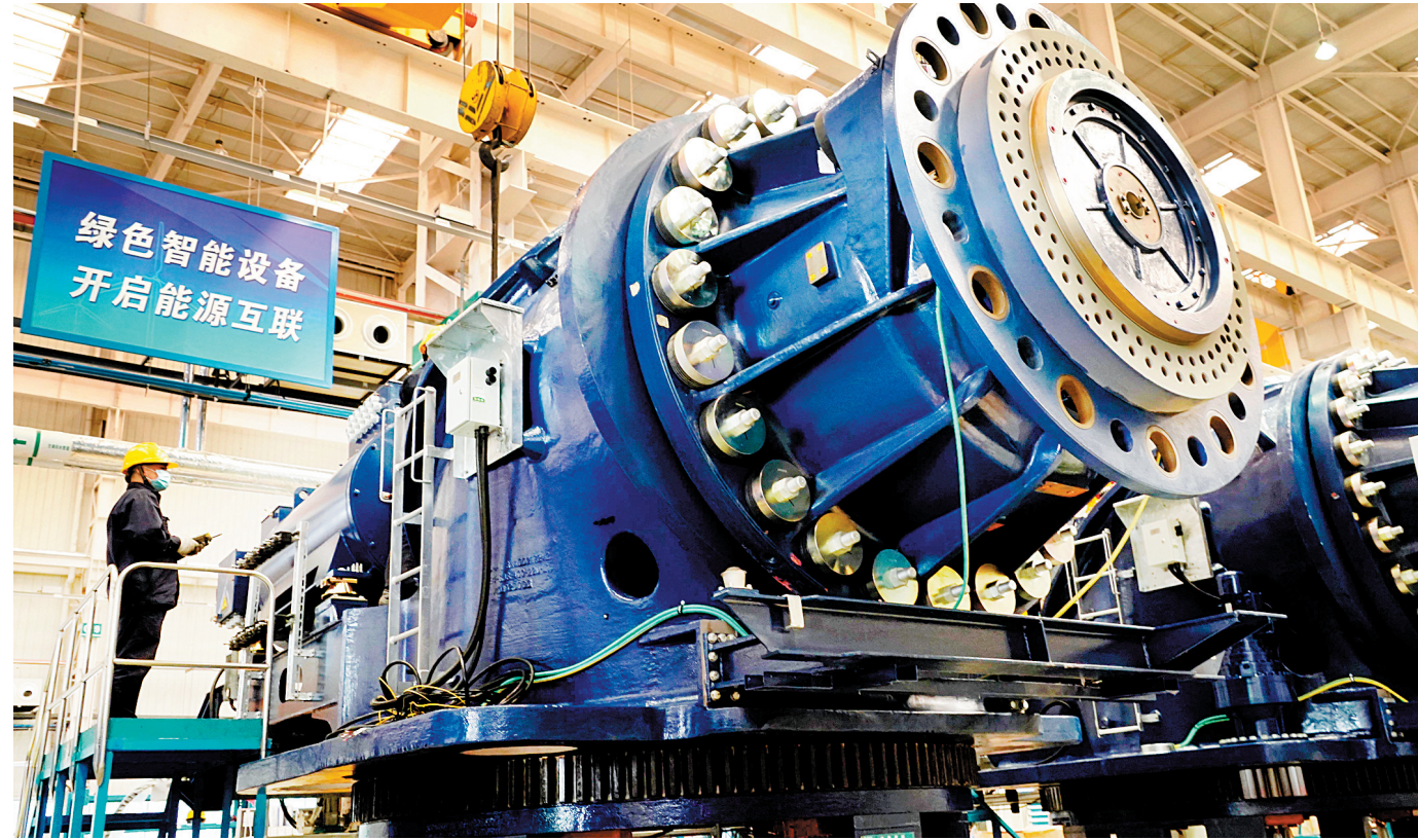
4月21日,工作人员在位于河南省许昌市的许继电气股份有限公司整机车间内作业(新华社记者 李安 摄)
